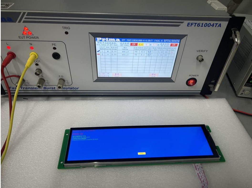
图 5-4 群脉冲测试图
