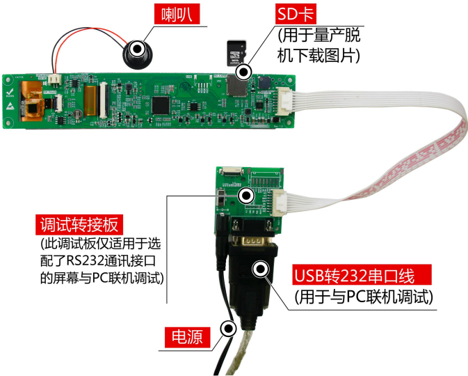
图 1-3 调试工具图
