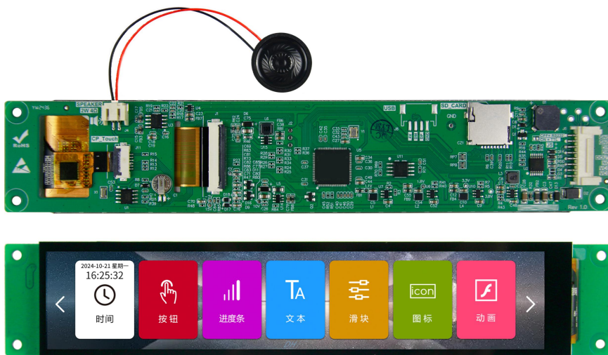
图 1-1 7.0 寸电容触摸参考图
