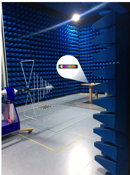
图 5-5 辐射测试图
